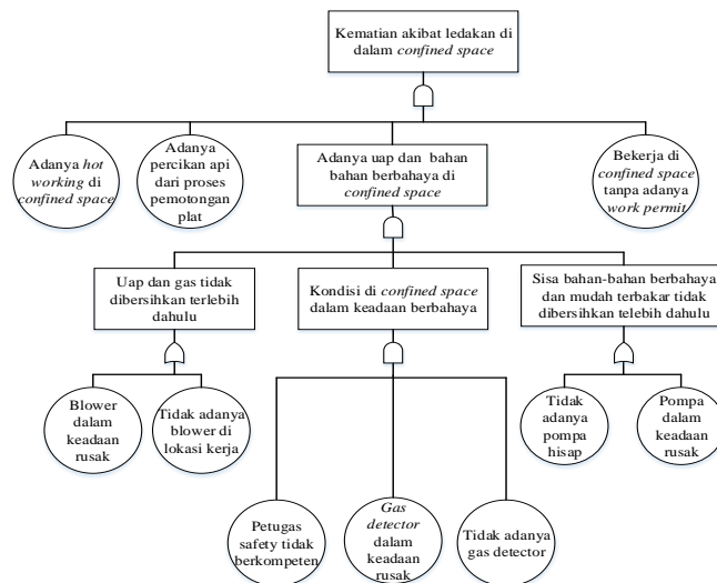
Gambar 2. Diagram FTA Kematian Akibat Ledakan di dalam Confined Space
