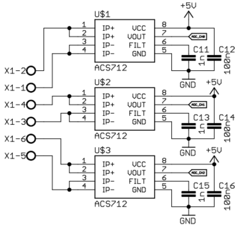
Gambar 2. Rangkaian Input Output Sensor Arus
