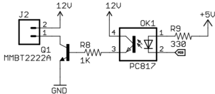
Gambar 3. Rangkaian Input Output Alarm
