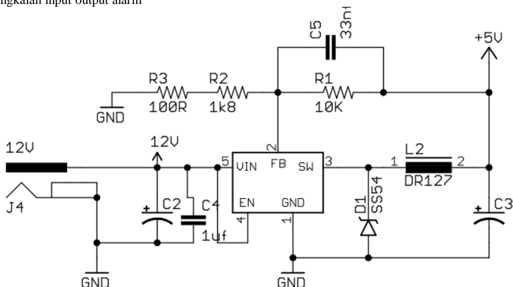
Gambar 1. Rangkaian Power
