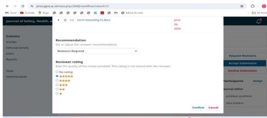
Gambar 17. Memberikan Rating
